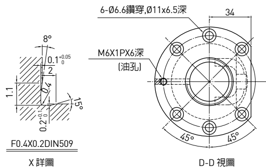
X 詳圖
