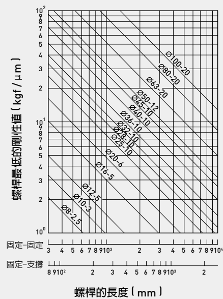
圖 4.29 螺桿剛性表
