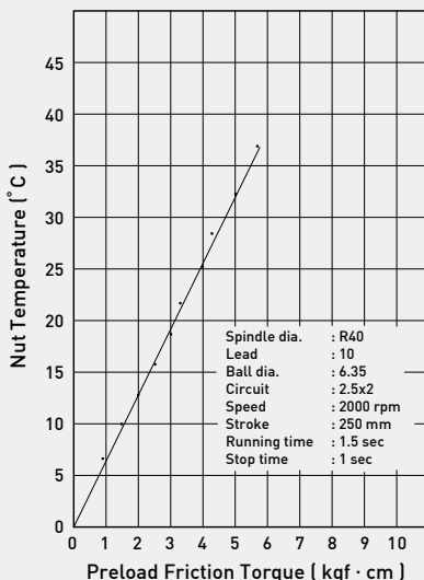
圖4.31 溫升與預壓摩擦扭矩的關係
