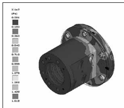
Cool Type滾珠螺桿的有限元素分析
