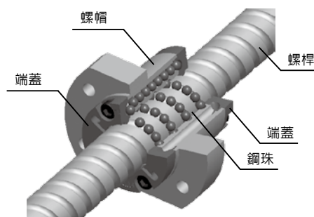
圖3.3 端蓋式滾珠螺桿
