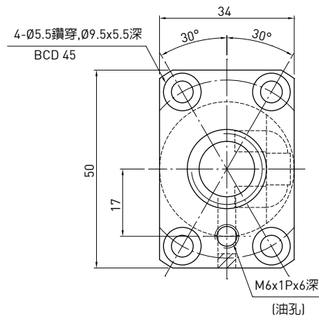
D-D 視圖
