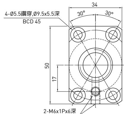
D-D 視圖
