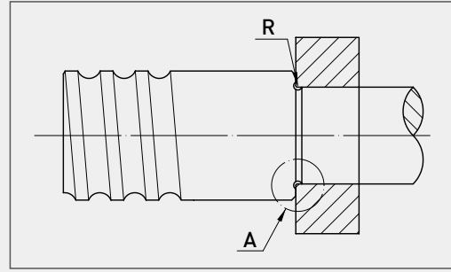
圖4.10 軸端承靠面的逃槽
