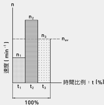
圖 4.22 等效速度
