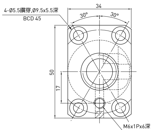
D-D 視圖
