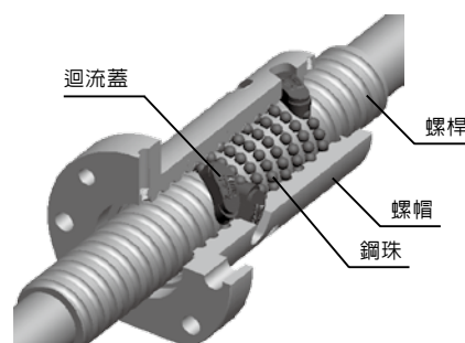
圖3.2 內循環滾珠螺桿
