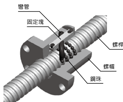
圖3.1 外循環滾珠螺桿
